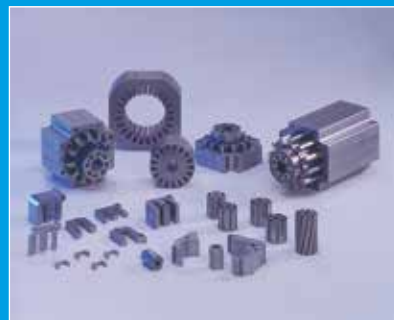
stanzpaketiert / pre-stacked
